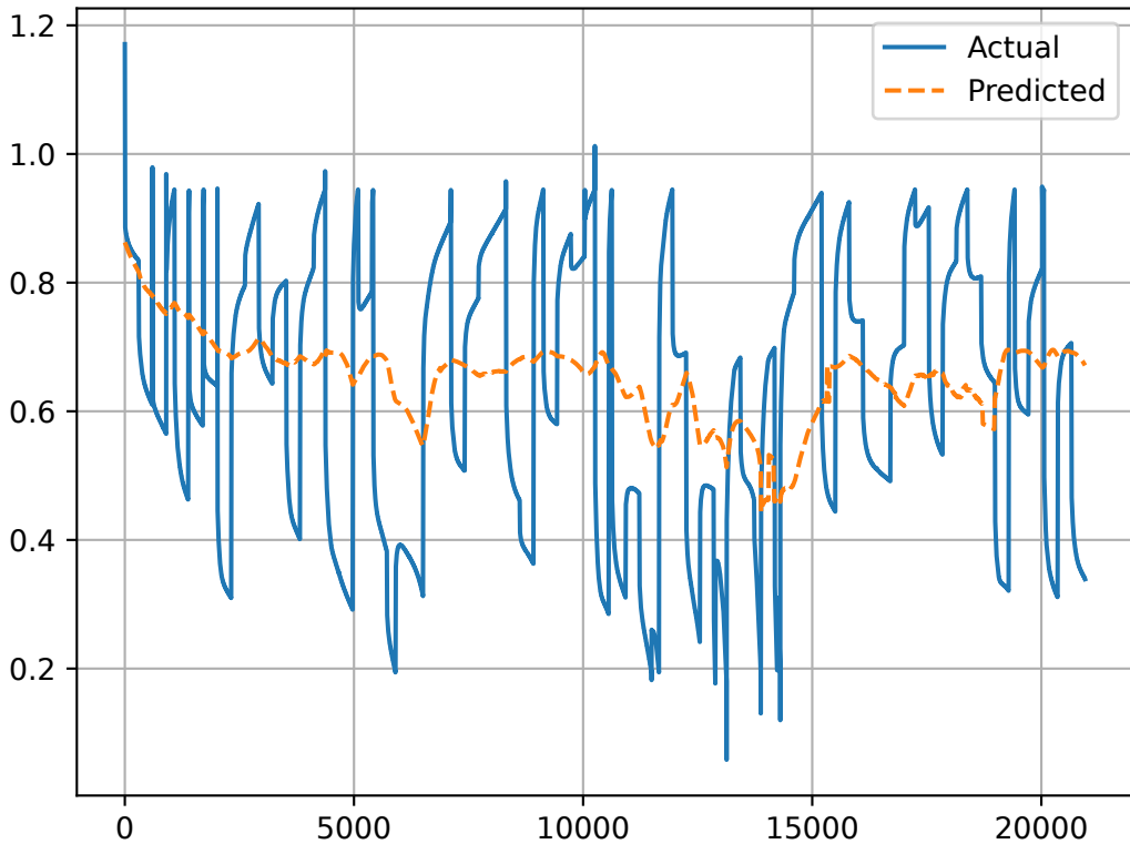
Predicted vs Actual (Test Set)
